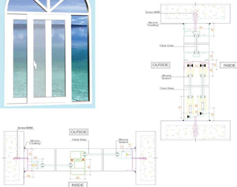
Cửa sổ lùa cố định trên hệ 70 Sliding window with top fixed frame series 70
