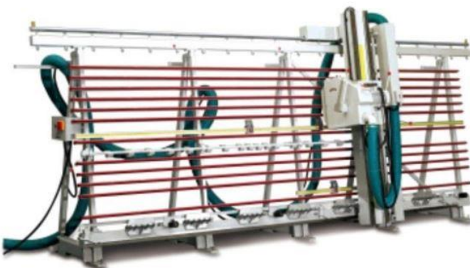
Máy cắt và khía tấm nhôm tổng hợp KT 971
