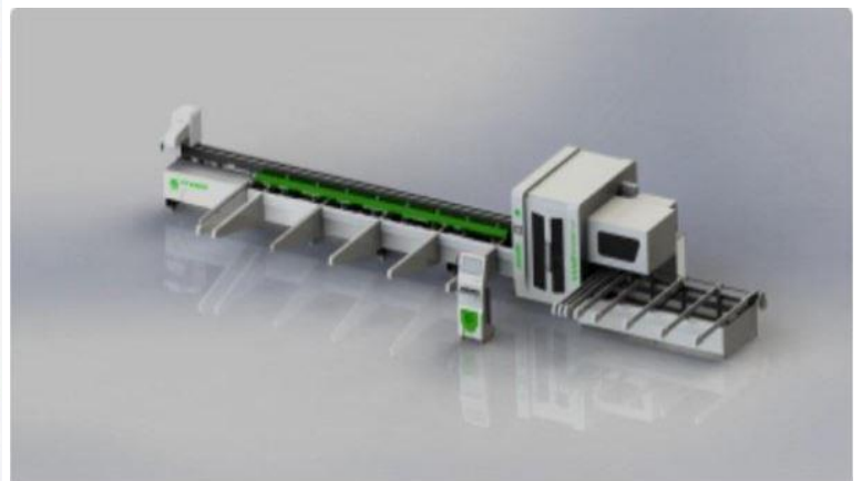
Máy cưa trung tâm CND 6000C
